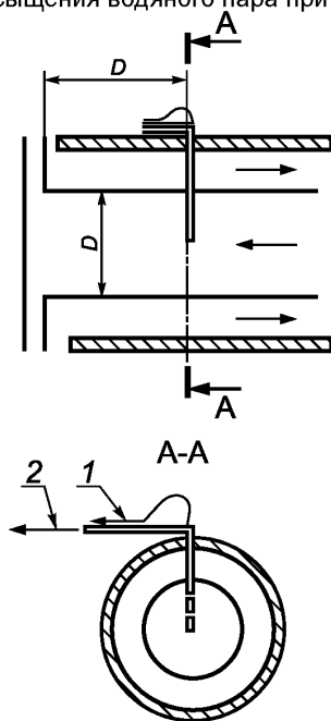
1 — к устройству для считывания температуры; 2 — к насосу для отбора проб
