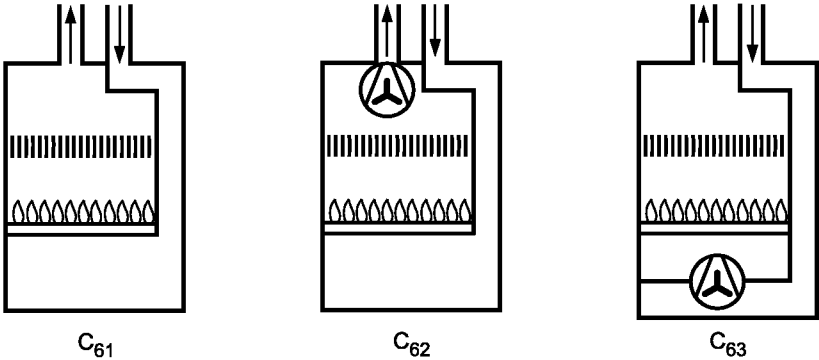
Рисунок В.6 — Схемы котлов типа C 6
