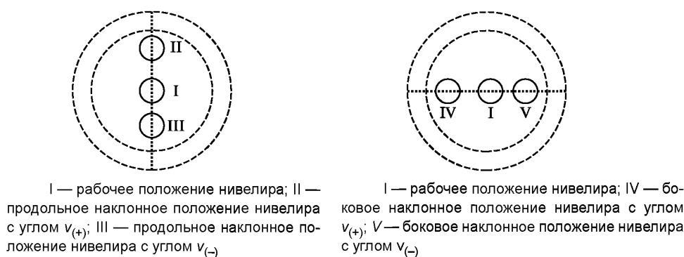
Рисунок 3 — Положения пузырька уровня при наклоне оси нивелира
