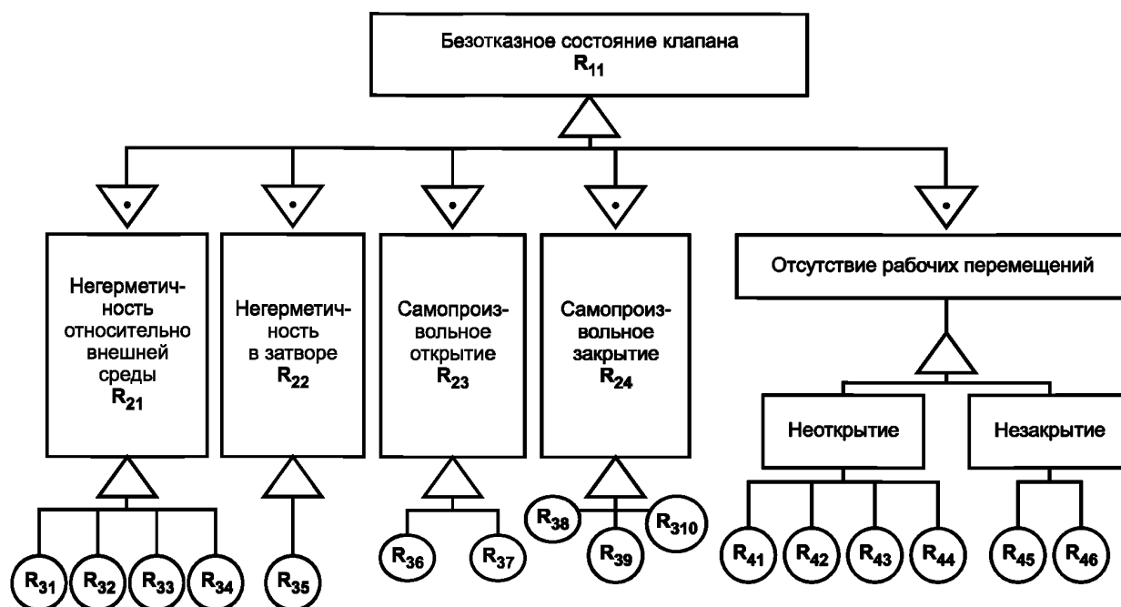
Рисунок A.8 — Схема отказов клапана
