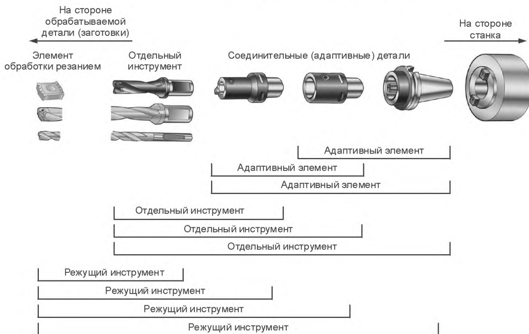
Рисунок 1 — Примеры разных типов сборок элементов
