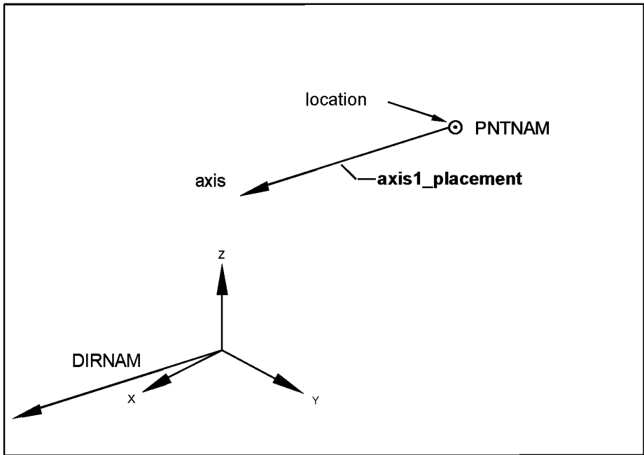
Location — размещение заданной точки; PNTNAM — опорная точка; axis — ось; axis1_placement — сущность axis1_placement ; DIRNAM — заданное направление
