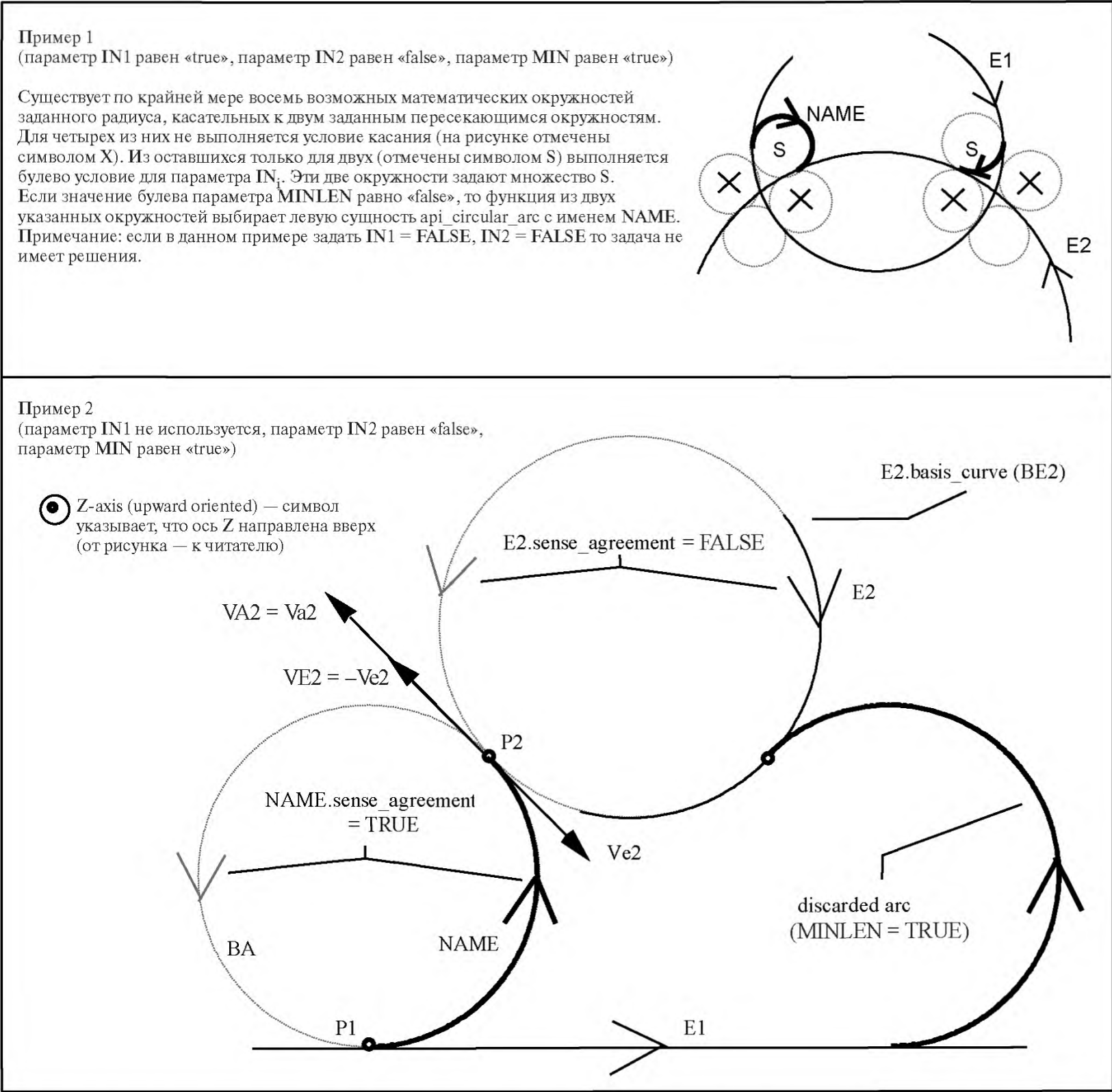
NAME — результирующая сущность; E2.basis_curve (BE2) — базовая кривая для исходной сущности E2 (BE2); E2.sense_agreement = FALSE — значение атрибута направления обхода сущности E2 равно «false»; NAME.sense_agreement = TRUE — значение атрибута обхода сущности равно «true»; discarded arc (MINLEN = TRUE) — исключенная дуга (значение параметра MINLEN равно «true»)
