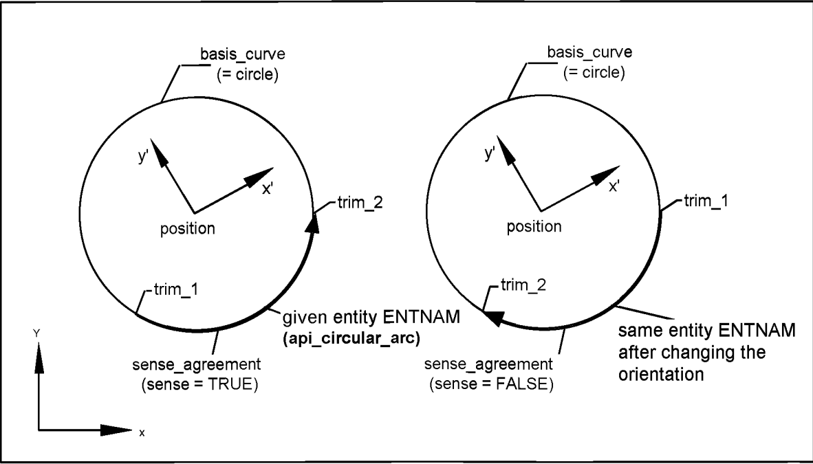
Basis_curve (= circle) — базовая кривая (окружность); trim_2 — вторая точка вычленения; trim_1 — первая точка вычленения; position — центр окружности; given entity ENTNAM (api_circular_arc) — исходная сущность ENTNAM (дуга окружности); same entity ENTNAM after changing the orientation — исходная сущность ENTNAM (дуга окружности) после смены положения; sense_agreement (sense = TRUE) — положительное направление обхода кривой; sense_agreement (sense = FALSE) — отрицательное направление обхода кривой
