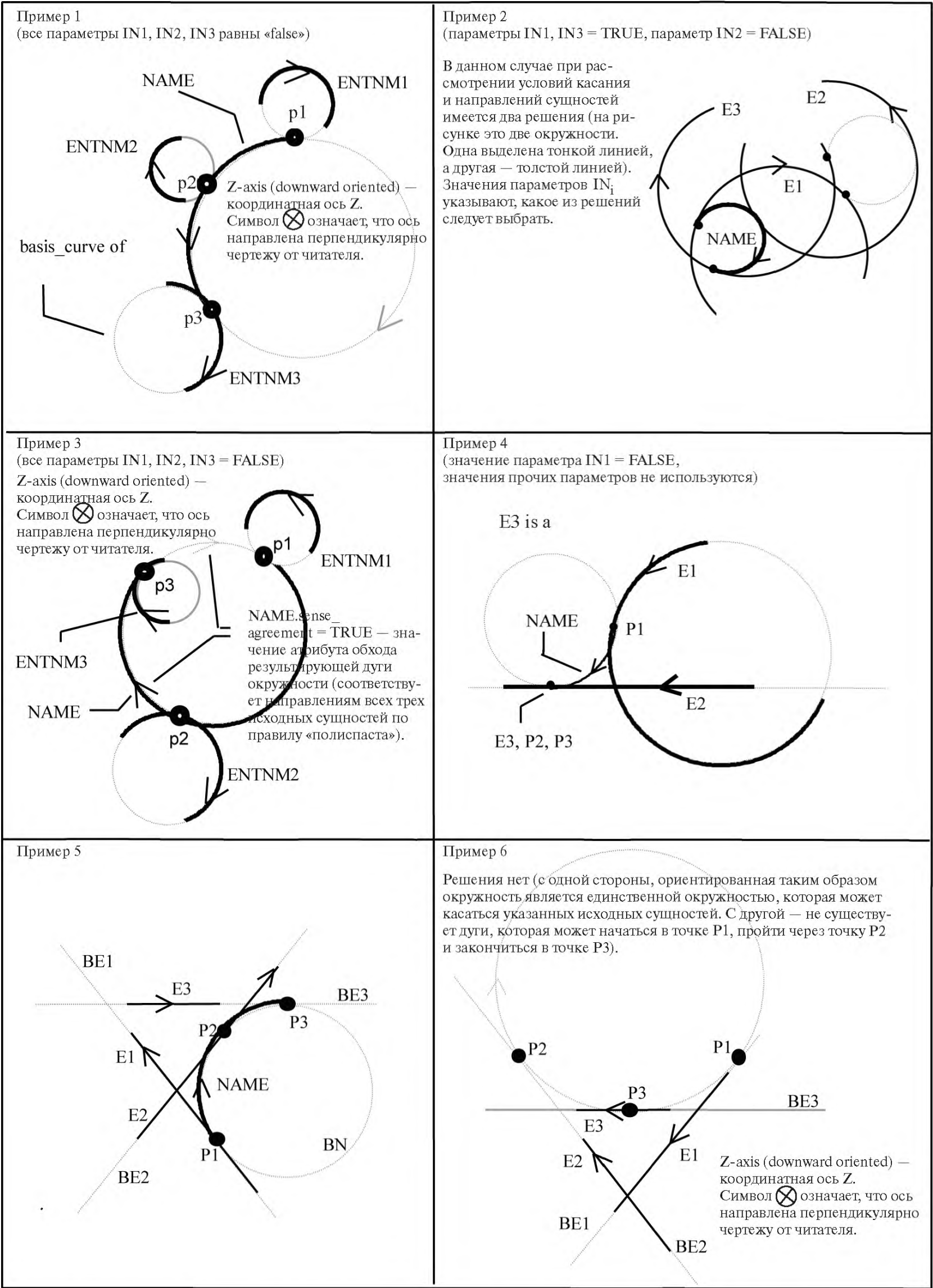
NAME — результирующая сущность (дуга окружности) NAME; ENTNM1 — исходная сущность (дуга окружности) ENTNM1; ENTNM2 — исходная сущность (дуга окружности ENTNM2); ENTNM3 — исходная сущность (дуга окружности ENTNM3); BE1 — базовая кривая (прямая) для исходного примитива E1 (также прямая); BE3 — базовая кривая (прямая) для исходной сущности E3 (также прямая); BN — базовая кривая (прямая) имени; BE2 — базовая кривая (прямая) для исходной сущности E2 (также прямая); E3 is a — исходная сущность E3 является декартовой точкой
