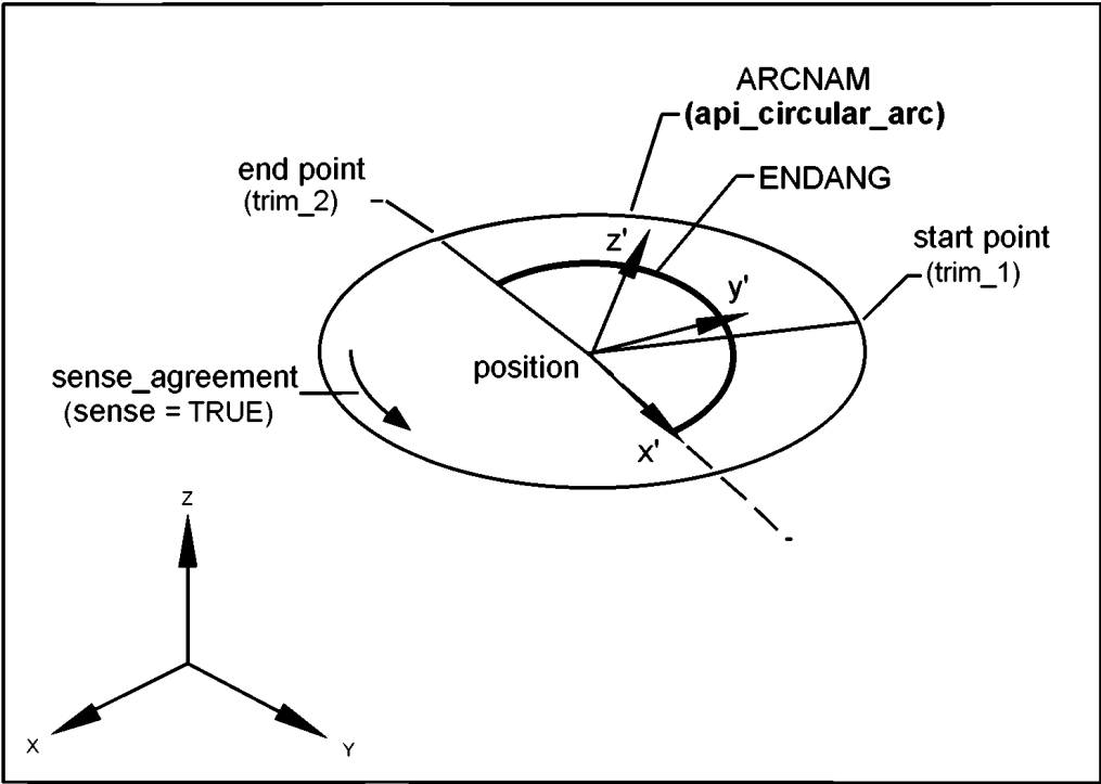
ARCNAM ( api_circular_arc ) — дуга окружности ARCNAM; end point ( trim_2 ) — конечная точка дуги (точка вычленения 2); ENDANG — конечный угол дуги окружности; start point ( trim_1 ) — начальная точка дуги (точка вычленения 1); position — центр окружности; sense_agreement ( sense = TRUE ) — положительное направление обхода кривой
