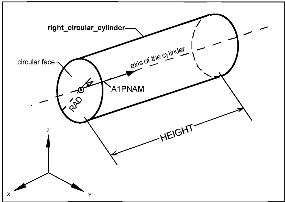
Right_circular_cylinder — прямой круговой цилиндр; axis of the cylinder — ось цилиндра; circular face — основание цилиндра; A1PNAM — локальная координатная система; RAD — радиус; HEIGHT — высота
