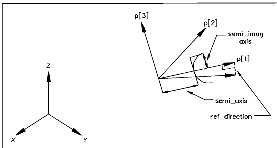
Semi_imag axis — мнимая полуось гипербола; semi_axis — действительная полуось гипербола; ref_direction — ссылочное направление
