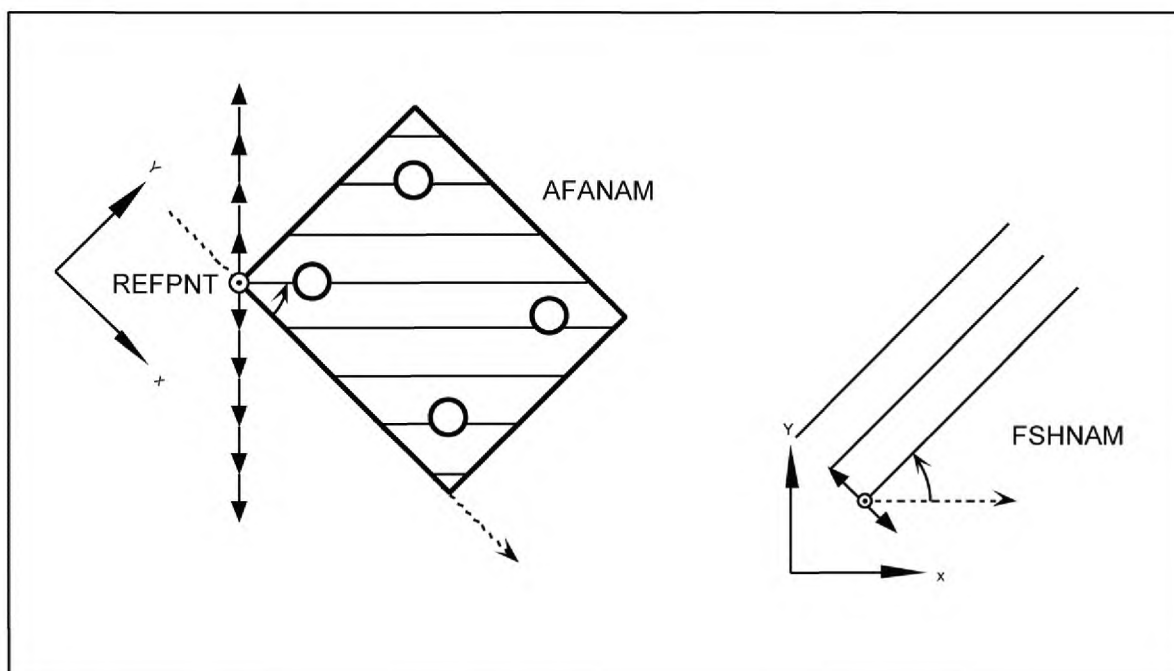
Рисунок А.37 — Функция Hatch_Afa
