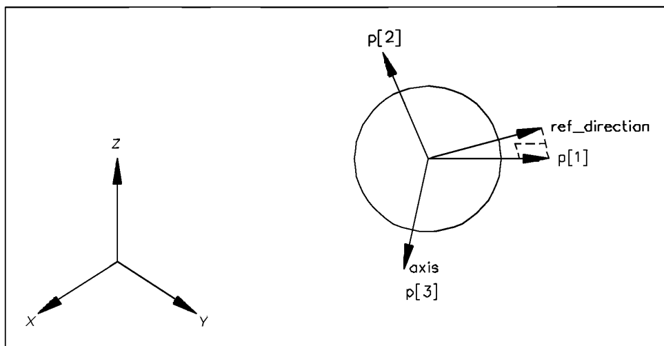
Рисунок 5 — Окружность
