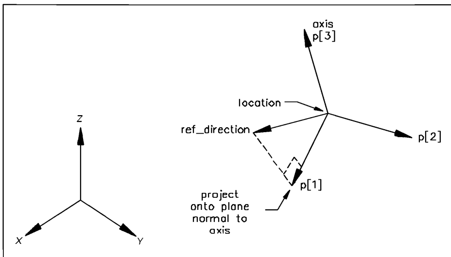
Рисунок 3 — Сущность axis2_placement_3D
