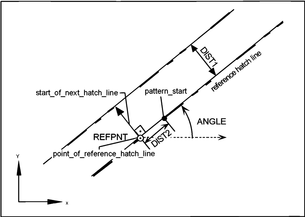
DIST1 — расстояние между линиями штриховки; reference hatch line — ссылочная линия штриховки; start_of_next_hatch_line — начало следующей линии штриховки; pattern_start — начало шаблона; ANGLE — угол наклона штриховки; REFPNT — ссылочная точка; DIST2 — расстояние от ссылочной точки до начала шаблона; point_of_reference_hatch_line — точка ссылочной линии штриховки
