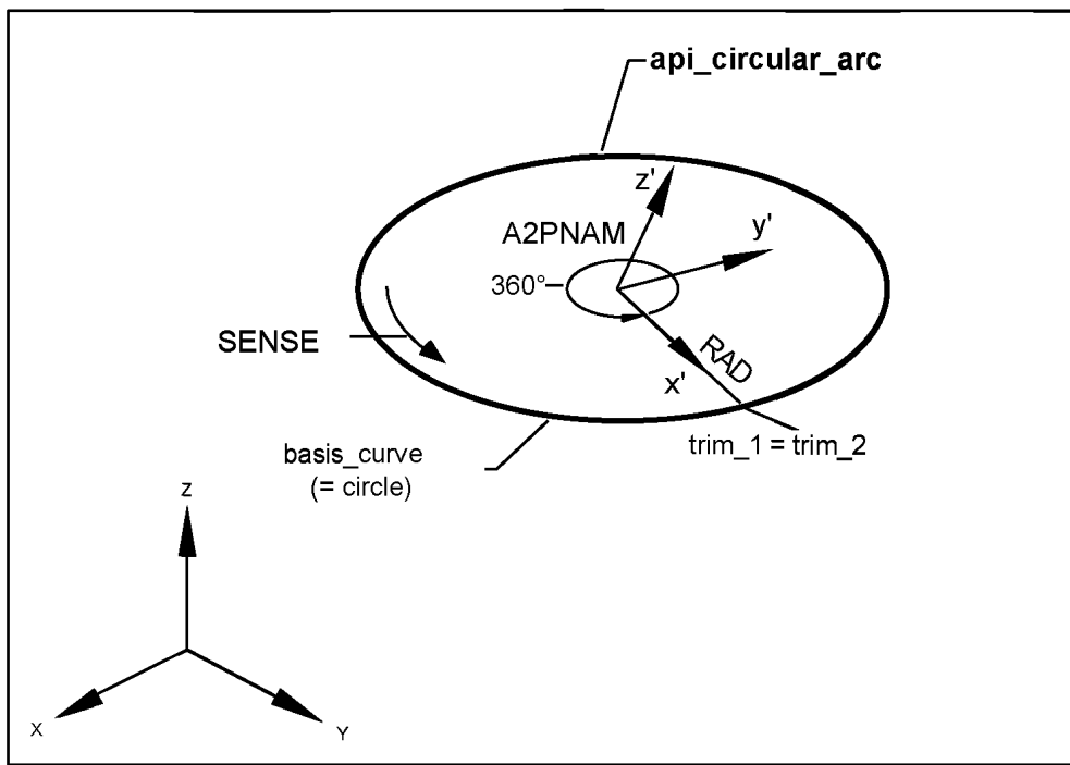
Api_circular_arc — построенная окружность; A2PNAM — центр окружности находится в начале локальной координатной системы; SENSE — положительное направление обхода окружности; RAD — радиус окружности; trim_1 = trim_2 — условие замкнутости окружности (начальная точка окружности совпадает с конечной точкой окружности); basis_curve (= circle) — базовая кривая (окружность)
