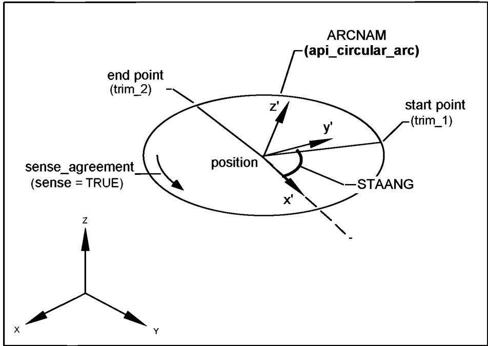
ARCNAME ( api_circular_arc ) — дуга окружности ARCNAME; end point ( trim_2 ) — конечная точка дуги (точка вычленения 2); start point ( trim_1 ) — начальная точка дуги (точка вычленения 1); sense_agreement ( sense = TRUE ) — положительное направление обхода кривой; position — центр окружности; STAANG — вычисляемый начальный угол дуги
