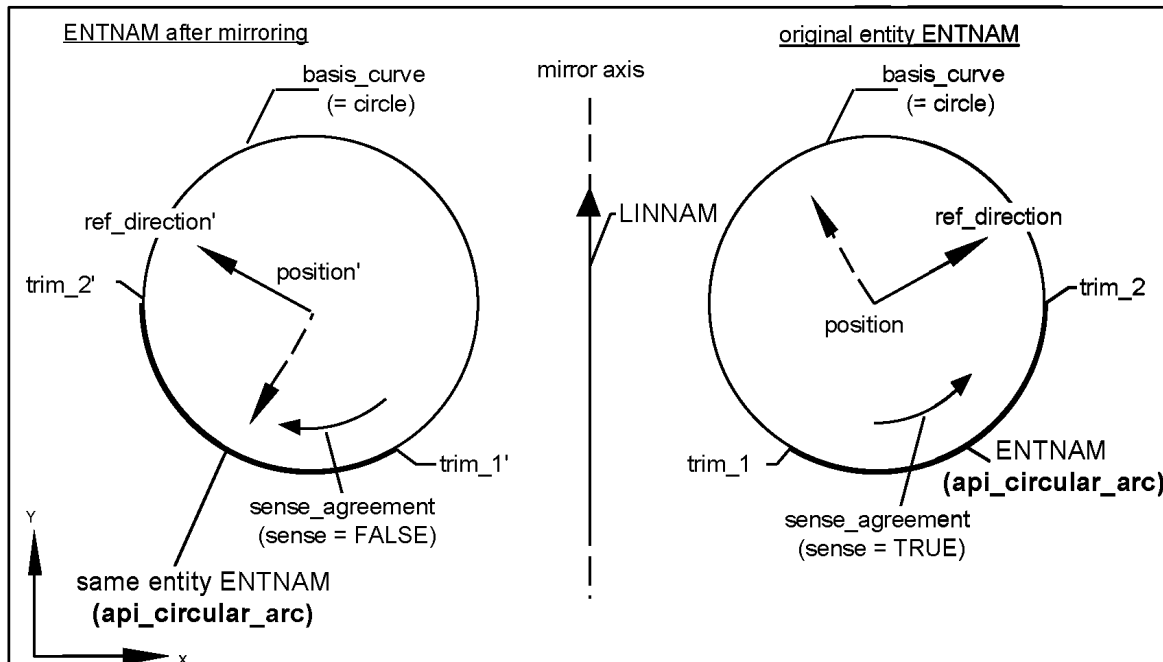
Рисунок А.50 — Функция Mirror_Ent (3D-вид)
