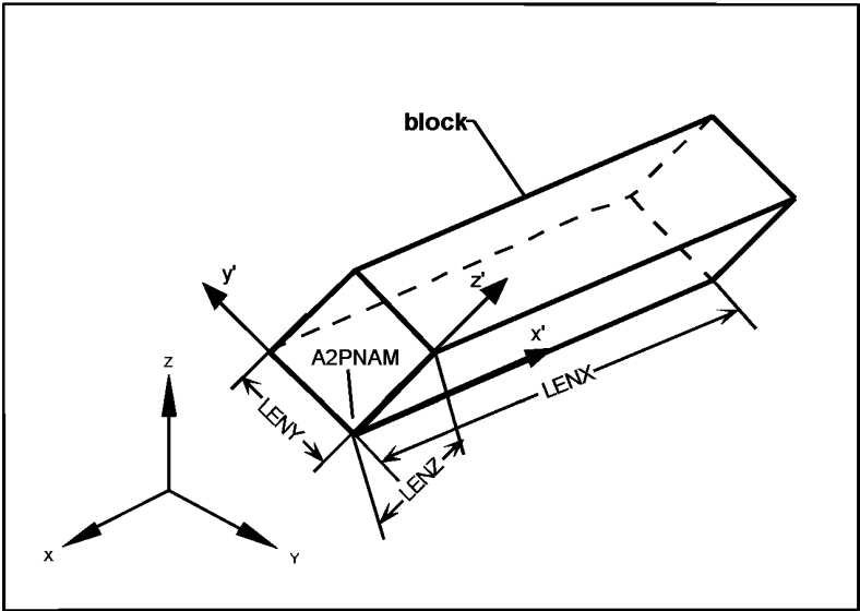
Block — блок; A2PNAM — имя локальной координатной системы; LENX — длина блока по оси X; LENY — длина блока по оси Y; LENZ — длина блока по оси Z
