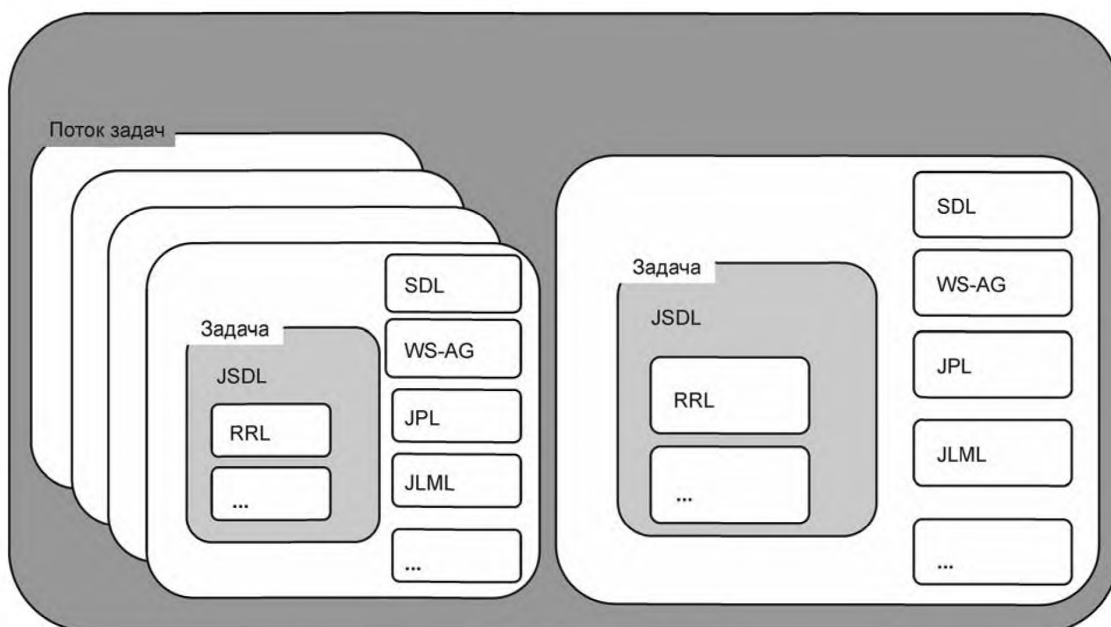
Рисунок 2 — Взаимодействие между JSDL и другими спецификациями
