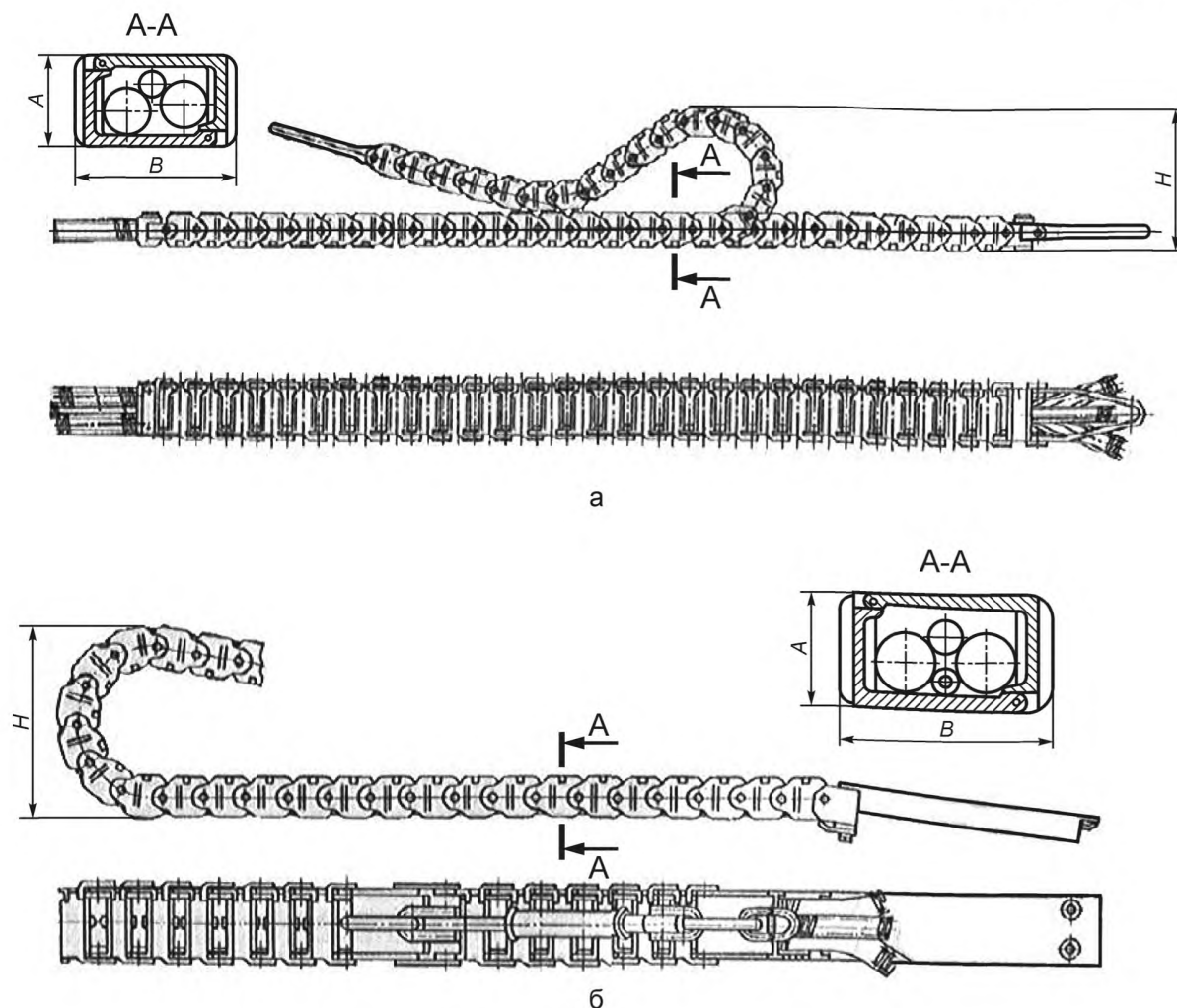
Рисунок 1 — Исполнение кабелеукладчика
