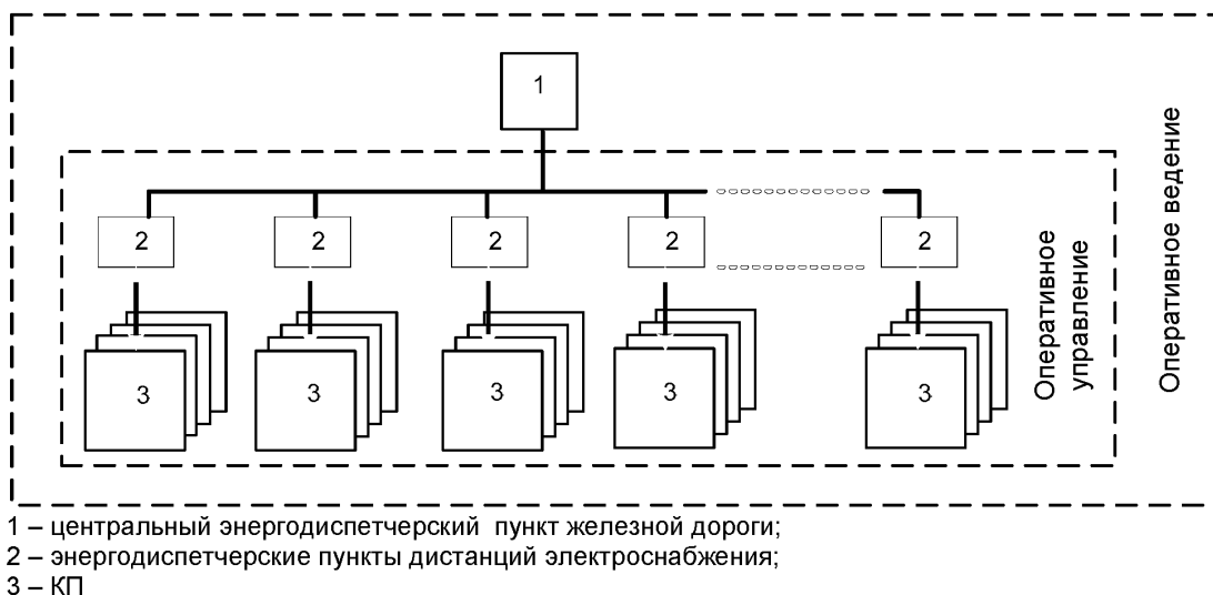
Рисунок 1 – Структура телемеханизации устройств электроснабжения железной дороги
