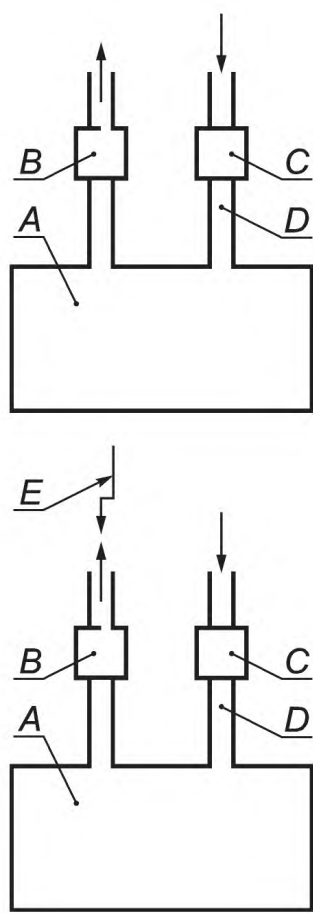
A — аппарат; B — место измерения давления; C — место измерения давления; D — пробоотборник для измерения CO 2 ; E — ограничитель
