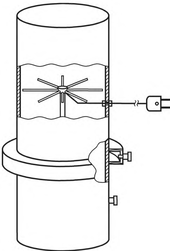
Рисунок 11 — Пробоотборник для аппаратов типа C 6
