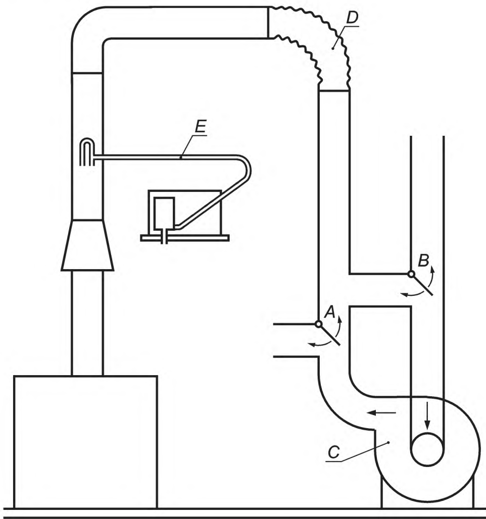
A, B — переключающие заслонки для обеспечения прямой и обратной тяги; C — вентилятор; D — гибкий патрубок; E — измерение скорости потока с помощью трубки Пито
