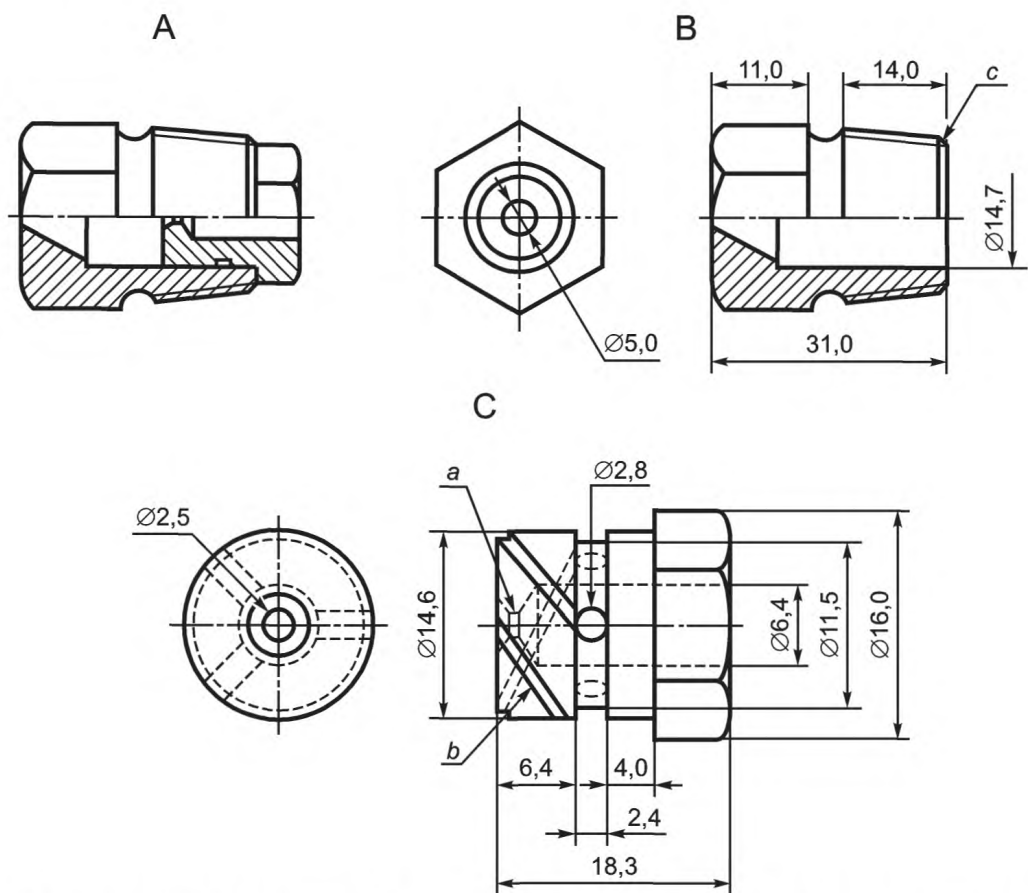
А — общий вид (сборочный узел); В — корпус; С — вставка; а — прямая шейка длиной 0,8 мм; сверление с углом раскрытия 115° глубиной 0,8 мм; b — три паза квадратным сечением 1,5 мм, глубиной 1,5 мм, с интервалом 120°, с углом наклона 60°, передняя кромка расположена по касательной к радиальной кромке; с — коническая резьба 1/2"
