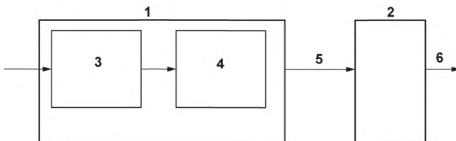
1 – EPSP; 2 – центральная группа; 3 – электронный датчик давления; 4 – преобразователь сигнала; 5 – интерфейс; 6 – разъем
