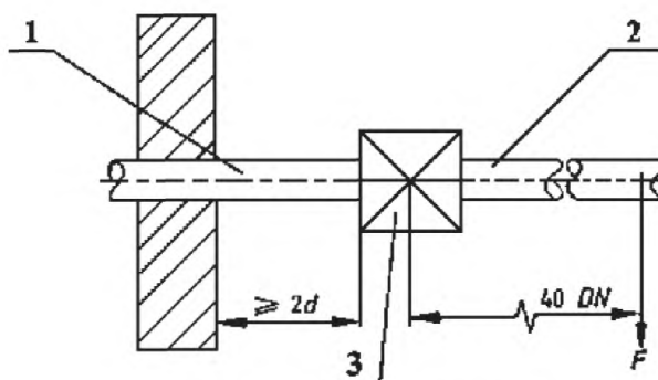
Рисунок 1 – Сборочный узел для испытаний регуляторов крутящим моментом
