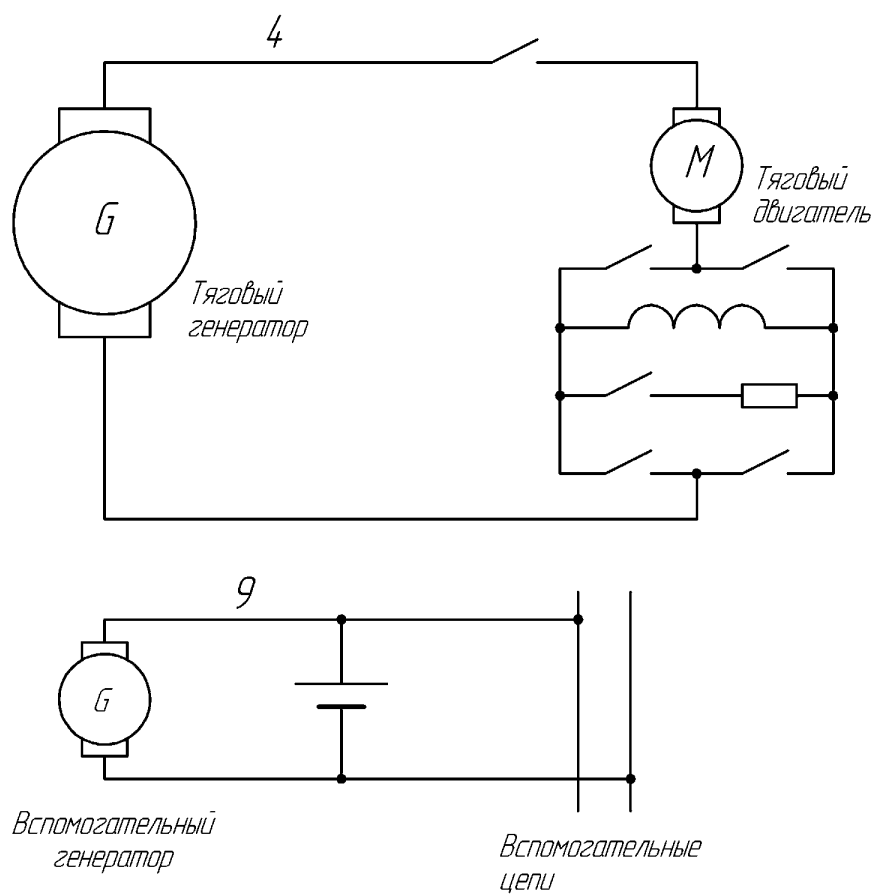
Рисунок А.5 – Система электропитания автономного железнодорожного подвижного состава с тяговым генератором и тяговым двигателем постоянного тока
