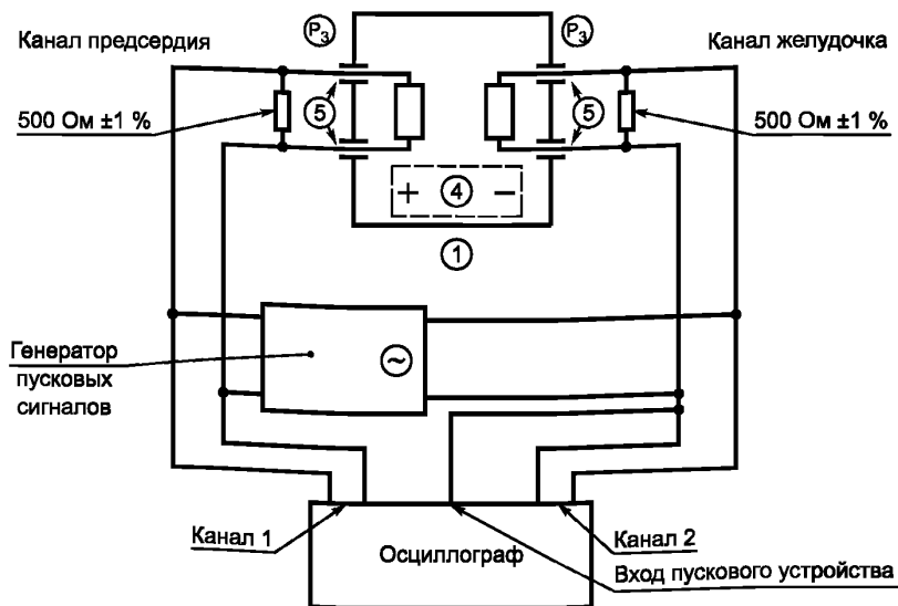
Объяснение к символам – по рисункам 10–27 общего стандарта. Рисунок 101 — Измерительная схема для МАКСИМАЛЬНОЙ ЧАСТОТЫ СЛЕЖЕНИЯ [см. 50.2 аа)]
