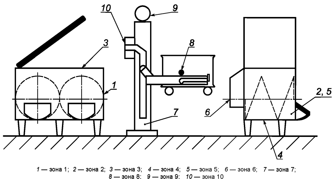
Рисунок 5 — Опасные зоны фаршемешалки
