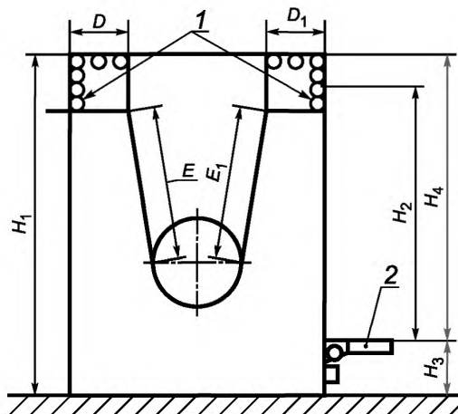
1 — перемещаемое защитное ограждение; 2 — блокирующая ступенька
