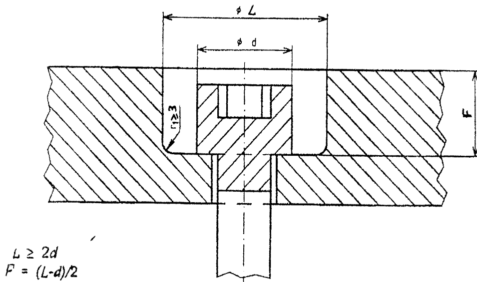
Рисунок А.4 — Пищевая зона. Винт с цилиндрической головкой и шестигранным углублением под ключ, вставляемый в опорную поверхность
