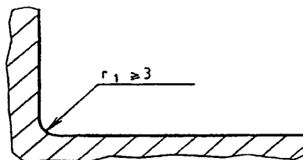
Рисунок А.1.1 – Пищевая зона. Закругленная кромка с радиусом, большим чем кривая с минимальным радиусом r_1 = 3 \text{ мм}
