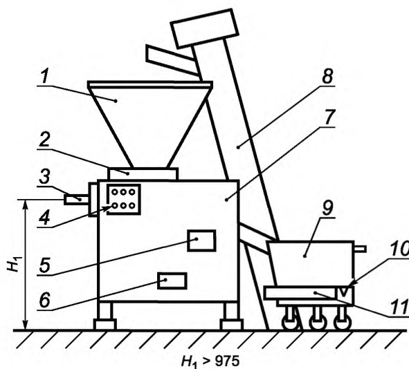
1 — питающий бункер; 2 — питатель; 3 — наполнительная цевка; 4 — выключатель «ВКЛ./ВЫКЛ.» с защитным колпачком; 5 — блокирующая ступенька; 6 — промежуточная ступенька; 7 — приводной механизм; 8 — загрузочное устройство; 9 — транспортная тележка; 10 — несущее устройство; 11 — подъемное устройство
