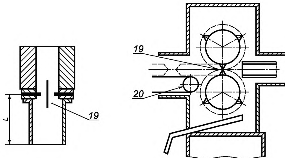
19 — зона 19; 20 — зона 20
