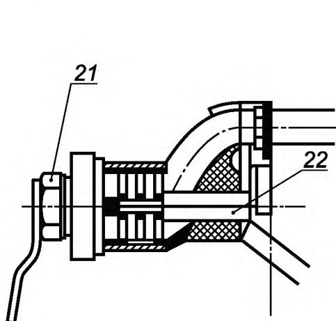
21 — зона 21; 22 — зона 22
