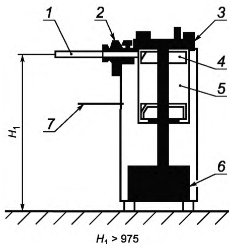
1 — наполнительная цевка; 2 — делительный поворотный кран; 3 — крышка цилиндра; 4 — поршень; 5 — цилиндр; 6 — приводной механизм; 7 — выключатель «ВКЛ./ВЫКЛ.» с защитным колпачком
