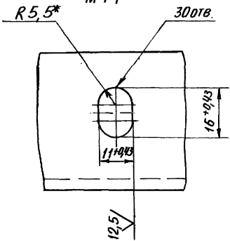
Вид А М 1:1
