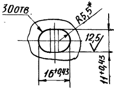
Вид Б М 1:1
