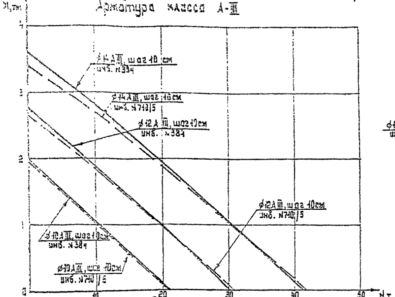
Графики несущей способности сечения по положительному моменту. Таблица расчетных характеристик сечения соединительной плиты
