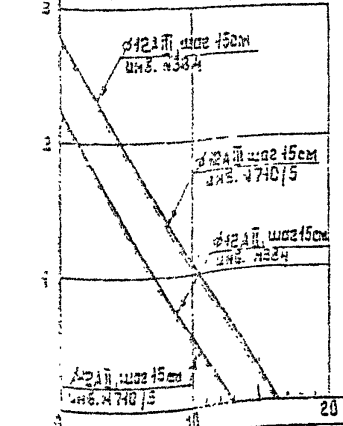
Графики несущей способности соединительной плиты. Таблица расчетных характеристик сечения соединительной плиты.
