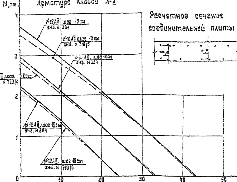
Графики несущей способности сечения по положительному моменту. Таблица расчетных характеристик сечения соединительной плиты
