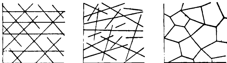
Рис. 1. Основные типы сетей трещин
