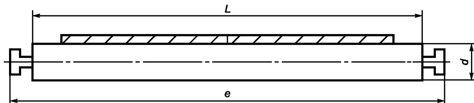
Рисунок 5 — Однороликовая опора
