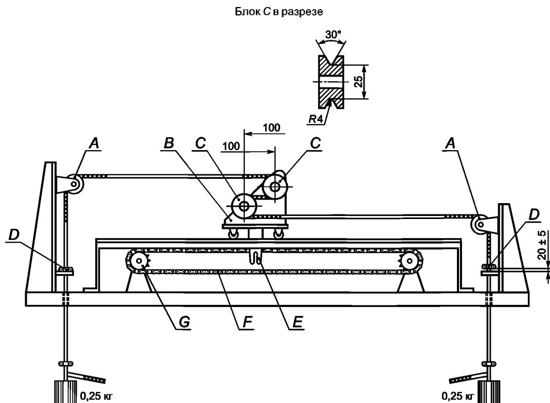
А — блок диаметром более 50 мм; В — тележка; С — блок с желобками; D — удерживающий зажим; Е — сцепляющий штырь; F — цепь с шагом 12,7 мм; G — зубчатое колесо с 20 зубчиками, диаметром начальной окружности 88,9 мм
