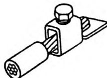
Контактный зажим с прямым прижатием жилы проводника
