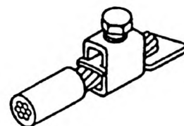
Контактный зажим с непрямым прижатием жилы проводника
