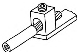
Контактный зажим с прямым прижатием жилы проводника
