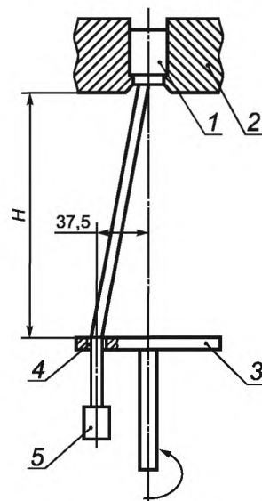
1 — зажим; 2 — подставка; 3 — плита; 4 — втулка; 5 — груз
