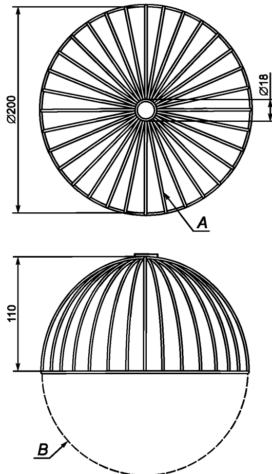
Рисунок 101 — Проволочный каркас
