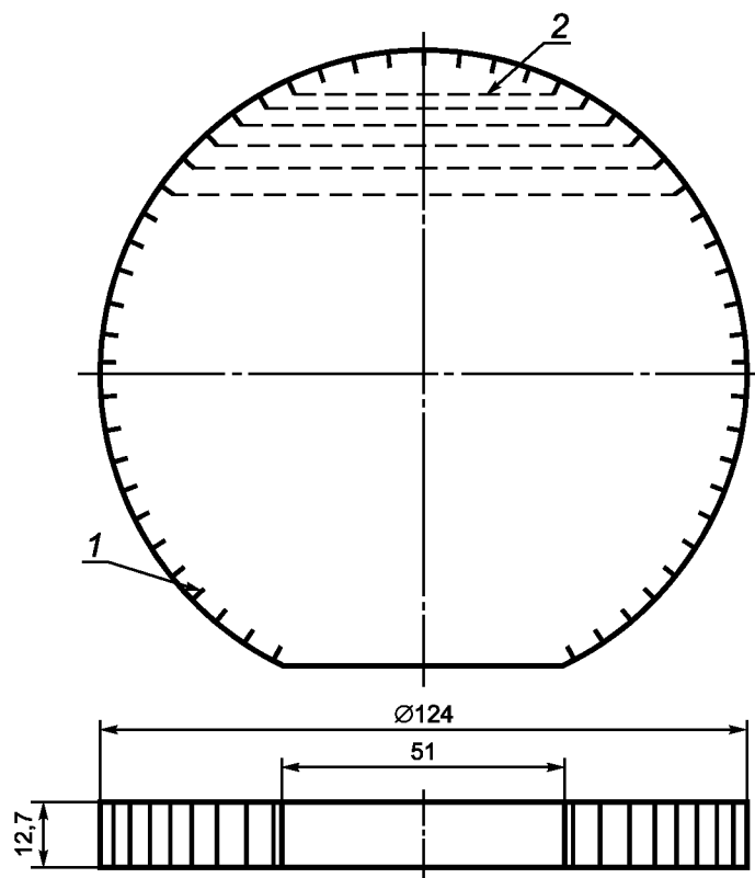
1 — паз размером 1,5 \times 1,5 мм на боковой поверхности диска; 2 — способ укладки никель-хромового провода диаметром 0,4 мм и длиной 2,5 м
