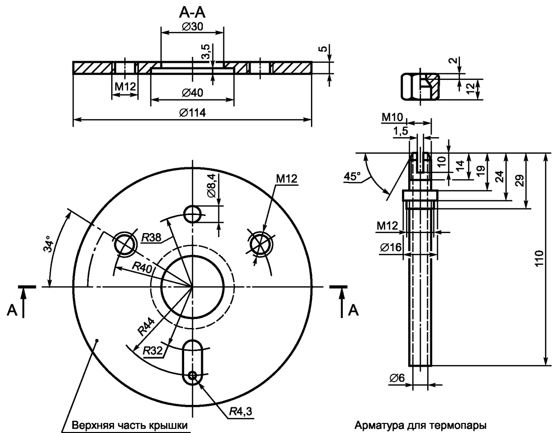
Рисунок А.8 — Крыка стального цилиндра
