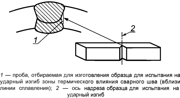
Рисунок 7 — Расположение образцов для испытания на ударный изгиб зоны термического влияния
