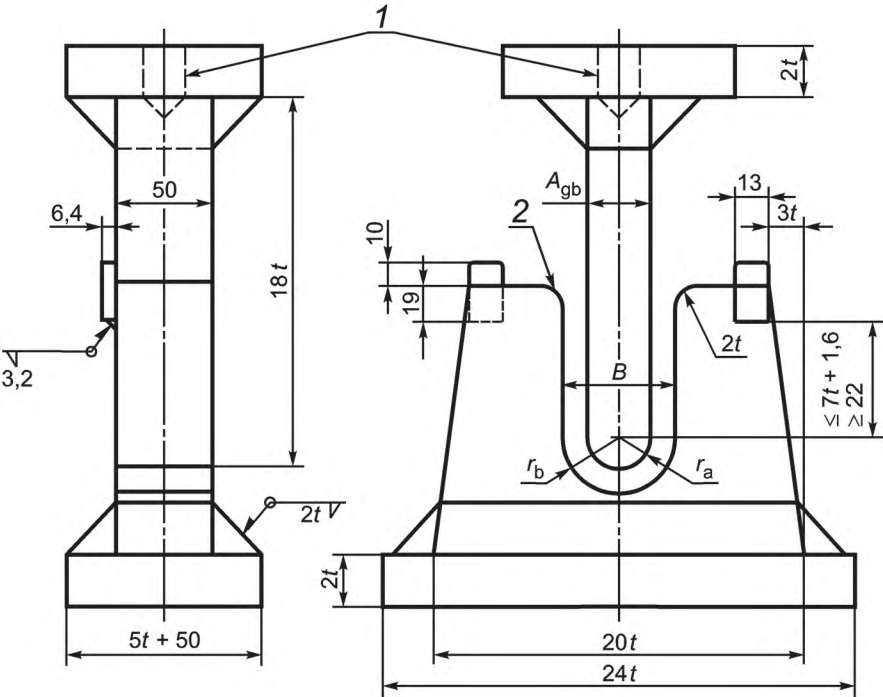
1 — резьбовое установочное отверстие; 2 — закаленные и смазанные опоры или закаленные ролики; B = A_{gb} + 2t + 3,2 мм; r_a — радиус оправки (пуансона) для испытания на направленный загиб; r_b — радиус матрицы для испытания на направленный загиб
