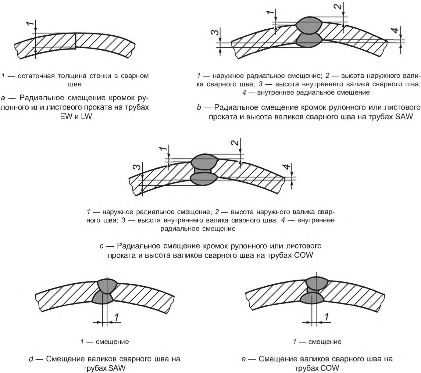
Рисунок 4 — Отклонения размеров сварного шва
