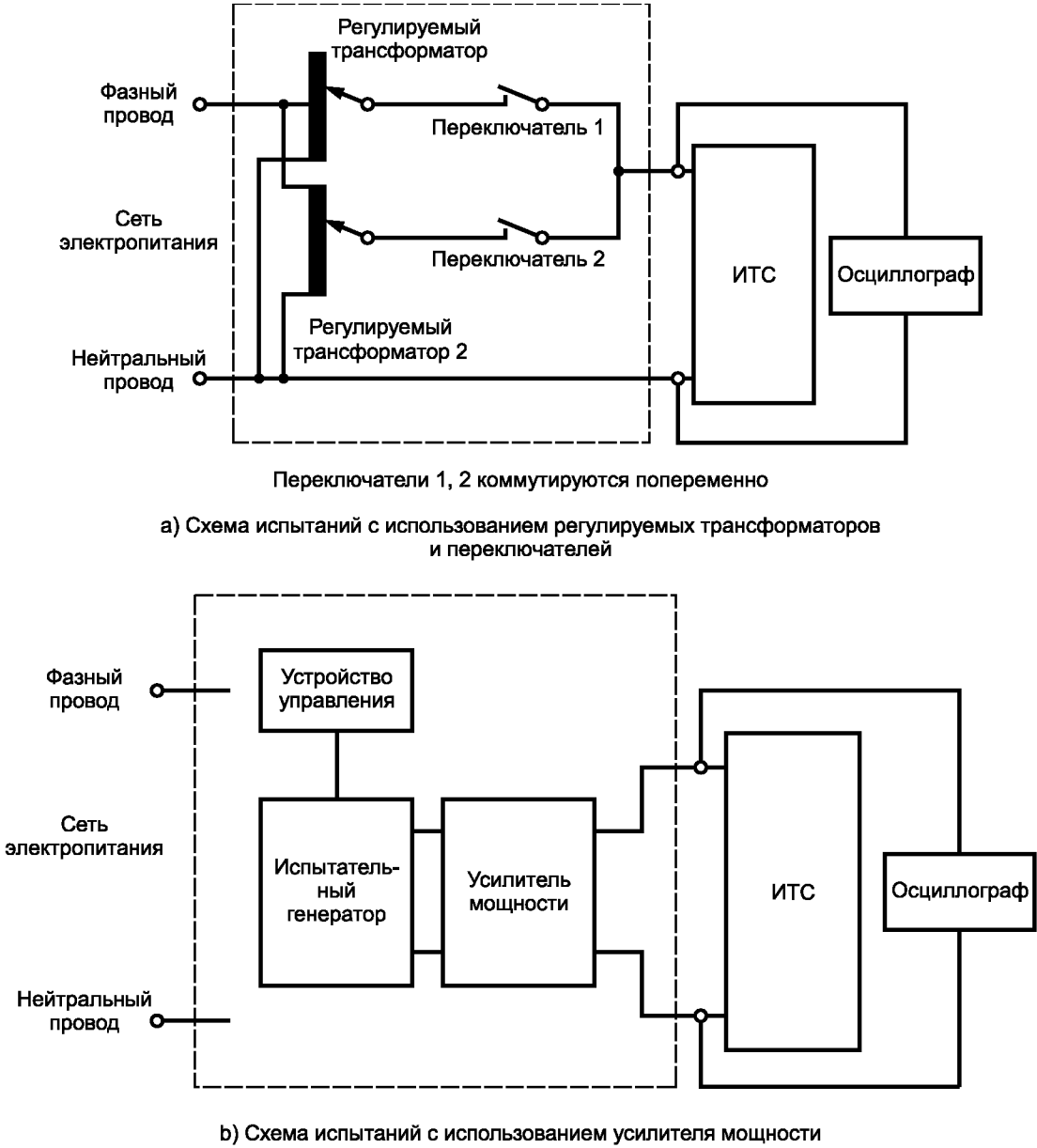
Рисунок С.1 — Схемы установок для испытаний при воздействии провалов, кратковременных прерываний и изменений напряжения электропитания, лист 1
