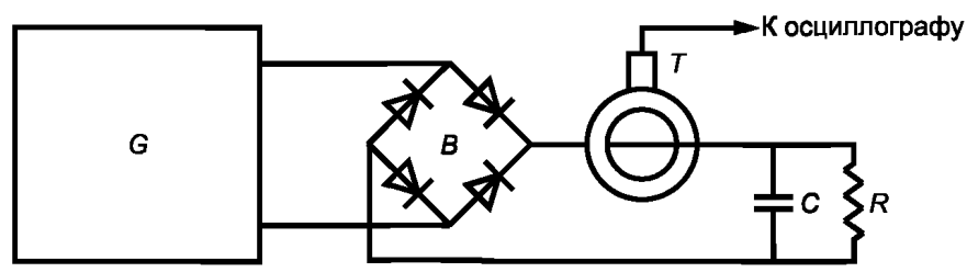
G — ИГ прерываний напряжения с переключением при 90^\circ и 270^\circ ; T — токосъемник; B — выпрямительный мост; R — резистор сопротивлением не более 10000\text{ Ом} и не менее 100\text{ Ом} ; C — электролитический конденсатор емкостью 1700\text{ мкФ} \pm 20\%
