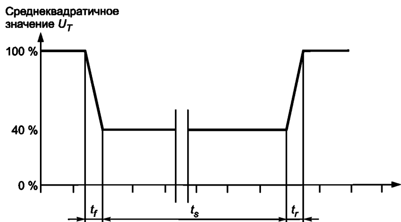
t_r — время нарастания напряжения; t_f — время понижения напряжения; t_s — время выдержки на пониженном напряжении
