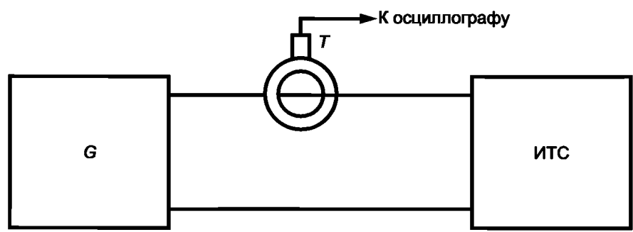
G — ИГ прерываний напряжения; T — токосъемник
