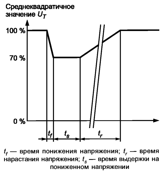
Рисунок 3 — Изменение напряжения
