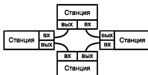
Рисунок 4 — Топология «кольцо»
