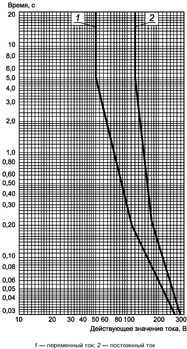
Рисунок С.1 — Кривая продолжительности предполагаемого напряжения прикосновения в соответствии с таблицей С.1
