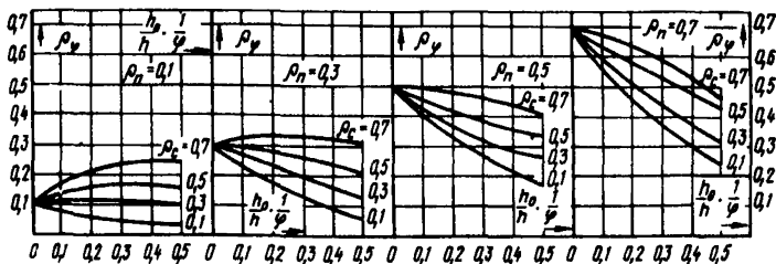
Рис. 44. График зависимости коэффициента отражения \rho_{\Phi} фиктивной плоскости от величины \frac{h_p}{h} \cdot \frac{\gamma}{\psi}
