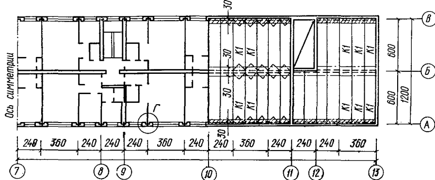
План этажа
