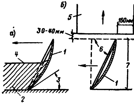
Рис. 4. Схема установки дискового плуга грейдер-элеватора
