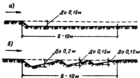
Рис. 3. Схемы резания грунта бульдозером а — прямоугольная; б — гребенчатая
