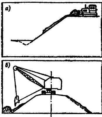
Рис. 7. Нанесение растительного грунта на откос
