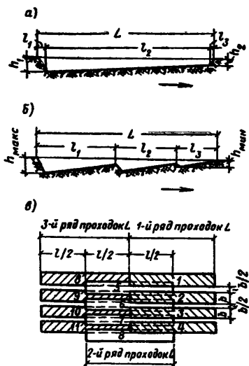
Рис. 2. Способы срезания грунта скрепером
