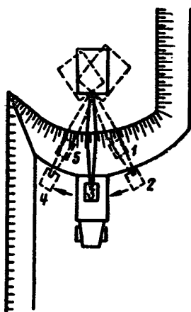
Рис. 1. Схема работы драглайна при загрузке грунтом автомобиля-самосвала челночным способом
