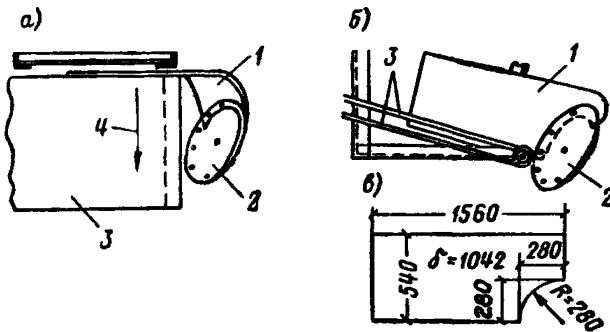
Рис. 5. Отражательный козырек грейдер-элеватора, служащий для уменьшения потерь грунта
