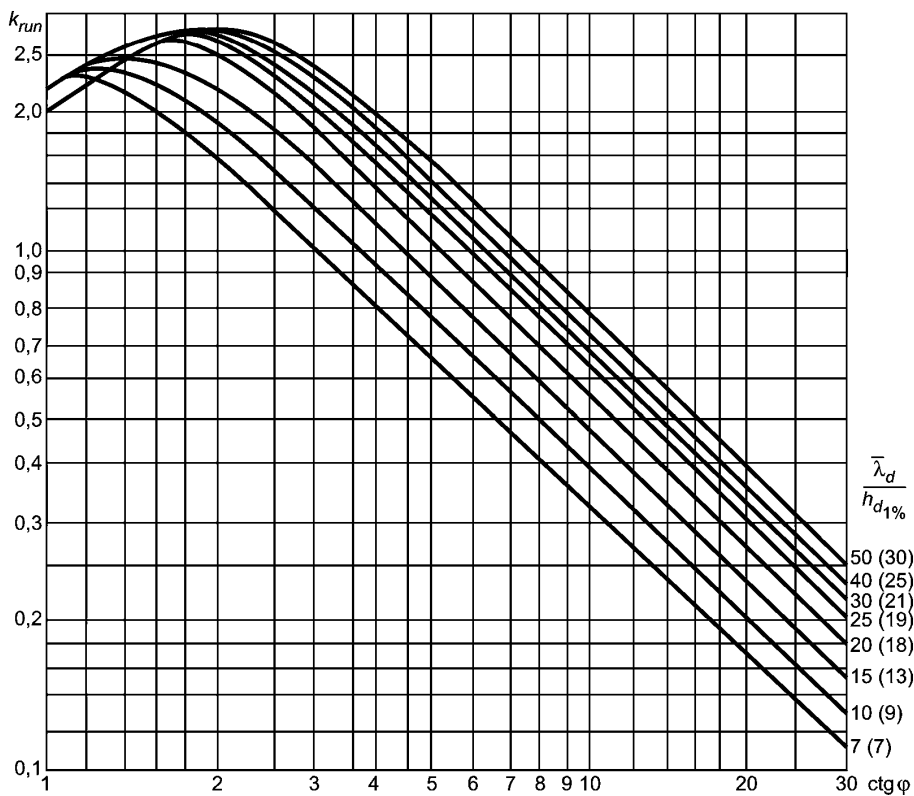
Рисунок 10 — Графики значений коэффициента k_{run}
