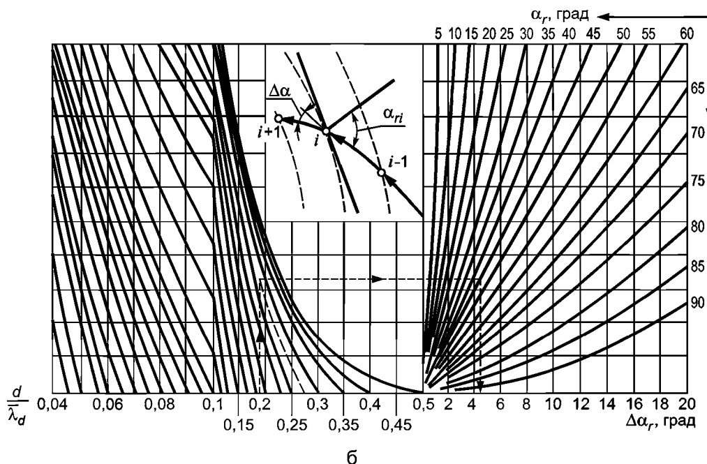
Рисунок А.6 — Схема (а) и графики (б) для построения плана рефракции
