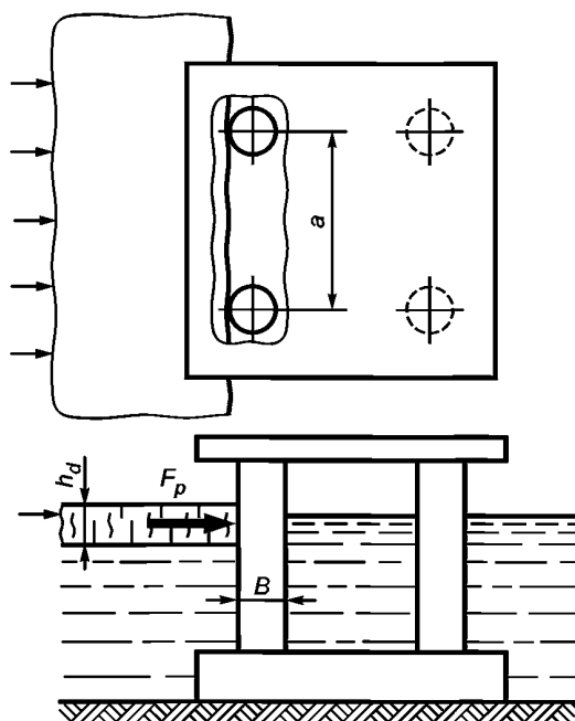
Рисунок 39 — Схема приложения нагрузок от движущегося ледяного поля на сооружение из системы вертикальных колонн
