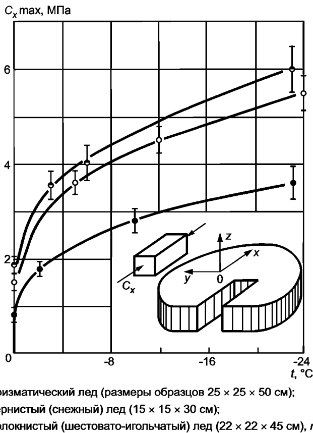
Рисунок Б.2 — Зависимость максимального предела прочности пресноводного льда при одноосном сжатии от температуры
