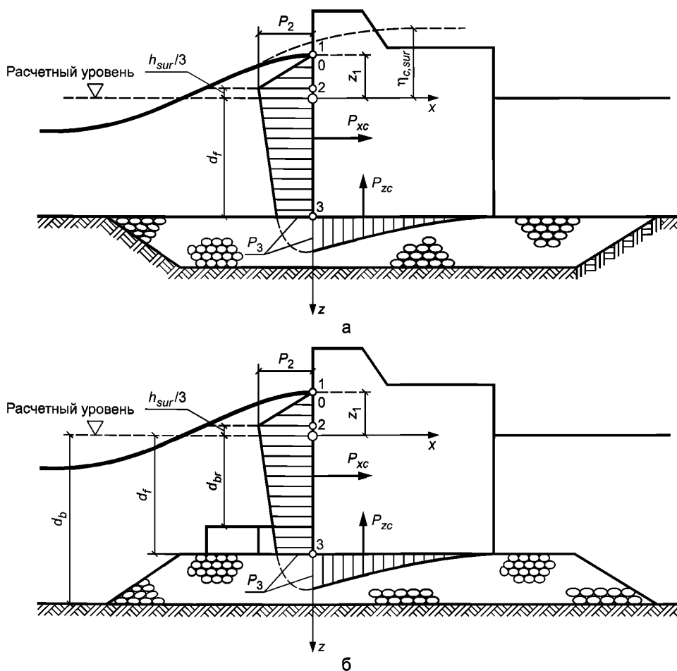
Рисунок 9 — Эпюры давления прибойных волн на вертикальную стену
