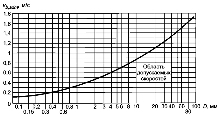
Рисунок 7 — График допускаемых значений неразрывающих донных скоростей
