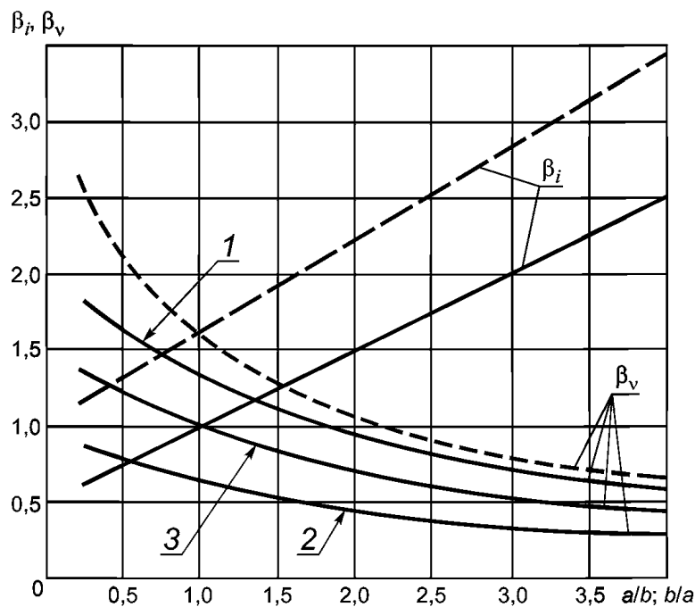
1 — для шероховатой эллиптической преграды; 2 — для гладкой преграды; 3 — для шероховатой в подводной и гладкой в надводной частях вертикальной эллиптической преграды
