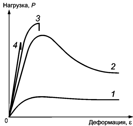
Рисунок Б.1 — Диаграммы «нагрузка — деформация» для льда, испытываемого при различных постоянных скоростях деформации: \dot{\varepsilon}_1 < \dot{\varepsilon}_2 < \dot{\varepsilon}_3 < \dot{\varepsilon}_4
