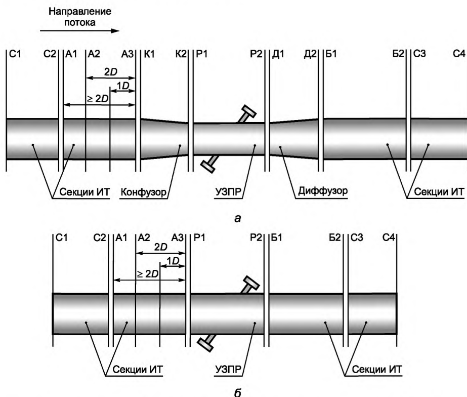
Рисунок 3 — Сечения ИТ, в которых выполняют измерения внутреннего диаметра в случаях: а — установки УЗГР с коническими переходами; б — установки УЗГР без конических переходов
