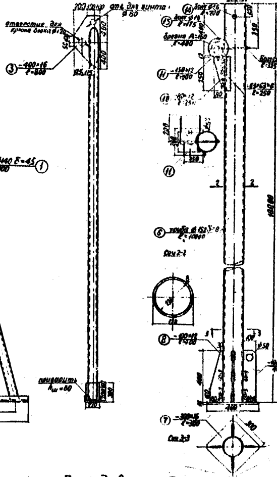
Рис. 4. Стальное оборудование для вывешивания дома
