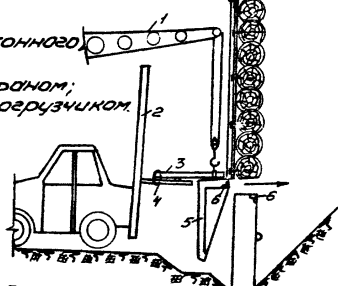
Рис.15. Монтаж цокольного элемента
