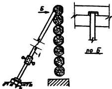
Рис. 2. Вывешивание осевого угла дамкратом с последующей фиксацией стен инвентарными подкосами: 1 - винтовой дамкрат на 10-15 т; 2 - металлический подкос; 3 - уголок.
