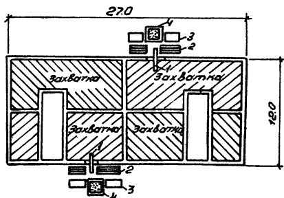
Рис. 19. План разбивки дома на захватки: 1 - кран "Волна" ДК-100, на чердачном перекрытии - кран "МК"; 2 - раскладка накладок для усиления балок и черепных брусьев; 3 - щиты наката; 4 - ящик с утеплителем (шлан, шлаковата и т.п.)
