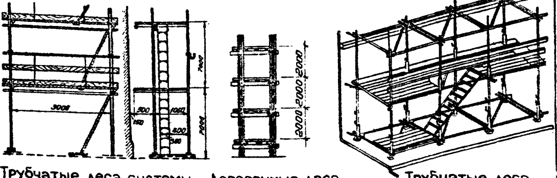
Деревянные леса системы Голобчинова
