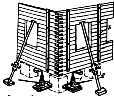
Рис. 2. Вывешивание осевого угла дамкратом с последующей фиксацией стен инвентарными подкосами: 1 - винтовой дамкрат на 10-15 т; 2 - металлический подкос; 3 - уголок.
