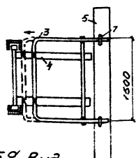
Рис.15а. Вид сверху на монтаж цоколя автопогрузчиком
