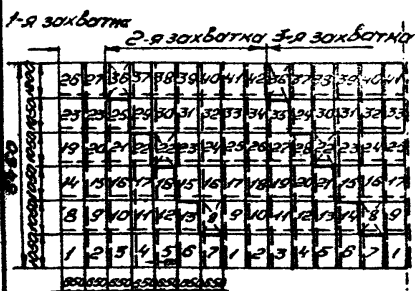
Рис. 40 а Пример разбивки площади ската кровли на захватки и очередность укладки листов при покрытии по методу Л.Т. Толстаго.
