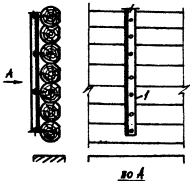
Рис. 3. Укрепление простенка уголком: 1 - инвентарный уголок.
