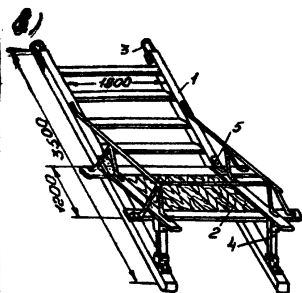
Инвентарная сборно-разборная площадка для приема волнистых листов на кровле:
