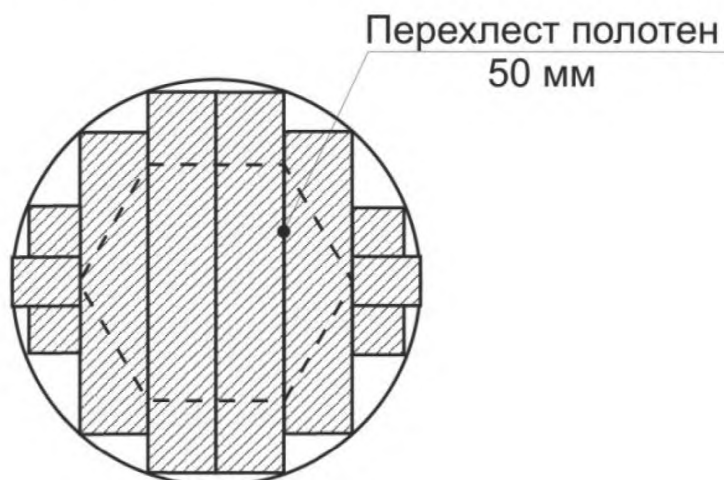
Рисунок А.3 – Раскладка стеклнных матов первого слоя
