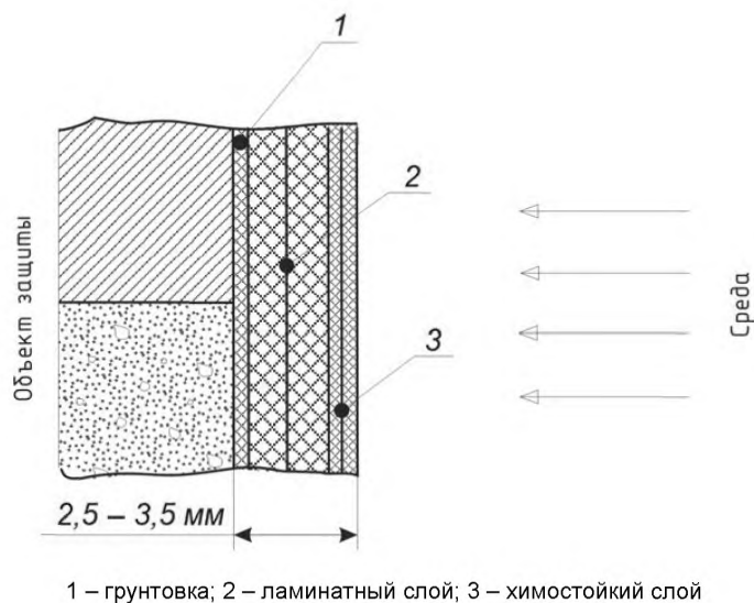
Рисунок 4.1 Общий вид футеровки
