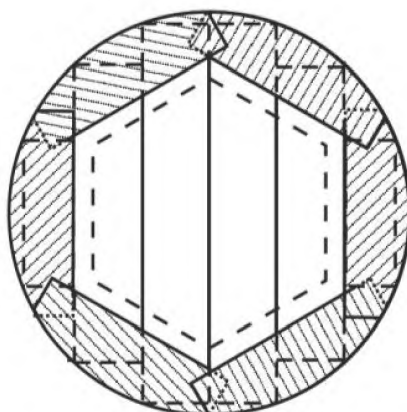
Рисунок А.4 – Раскладка стекляных матов второго слоя в примыканиях
