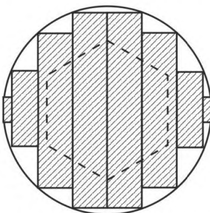
Рисунок А.5 – Раскладка стекляных матов второго слоя
