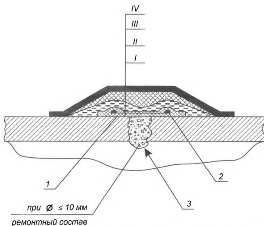
I – специальный слой; II – технологический слой; III – силовой слой; IV – защитный слой; 1 – накладка; 2 – биндаж; 3 – сквозное повреждение Рисунок 8.3
