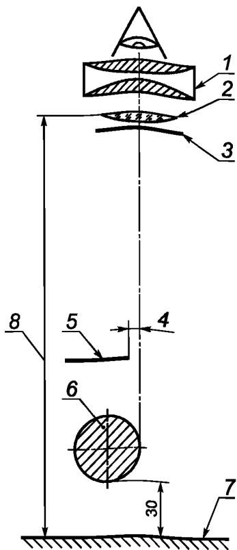
1 — увеличительное устройство; 2 — контактная линза; 3 — опора для контактной линзы; 4 — регулируемая ширина освещенного участка; 5 — диафрагма; 6 — люминесцентная лампа; 7 — матовая черная пластина:150 мм × 360 мм; 8 — контрольное расстояние: 400 мм
