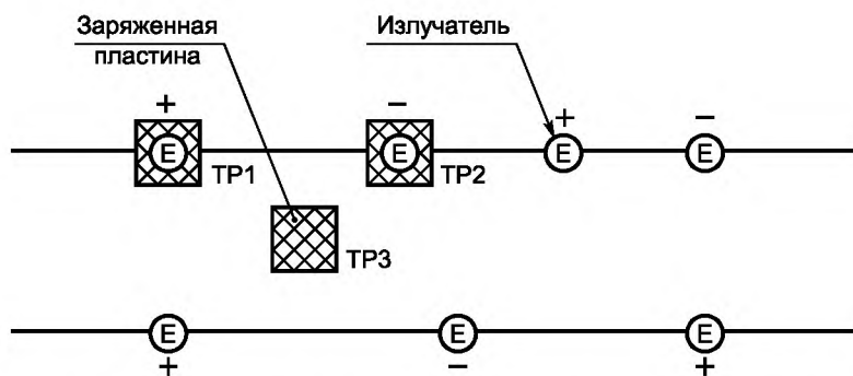
Рисунок 5. Области испытаний ионизации всего помещения. Системы двояных линий постоянного тока
