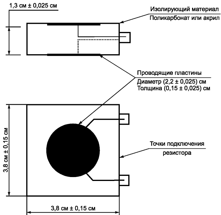
Рисунок 2 — Плоскопараллельный емкостный зонд
