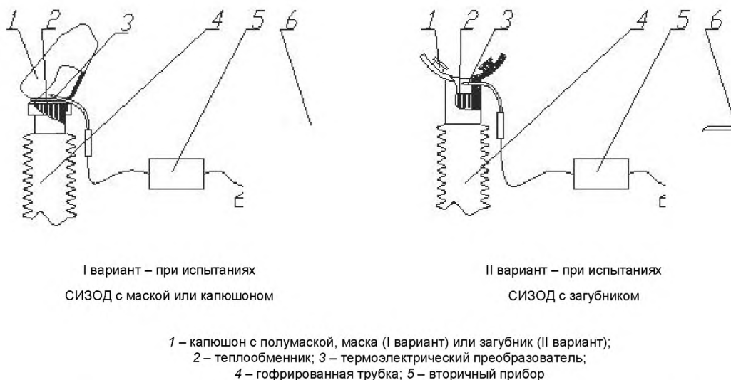
Рисунок 1 – Принципиальная схема измерения температуры вдыхаемой ГДС
