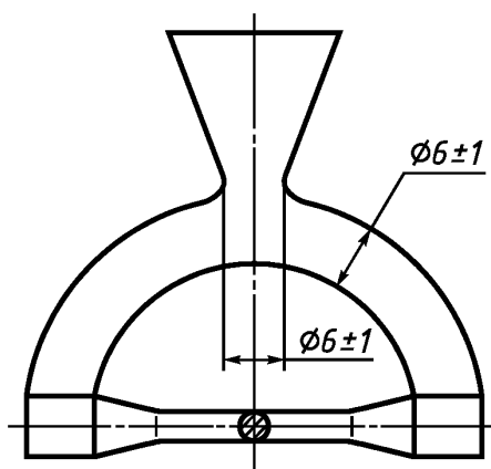
Рисунок 4 — Образец с рекомендуемой литниковой системой
