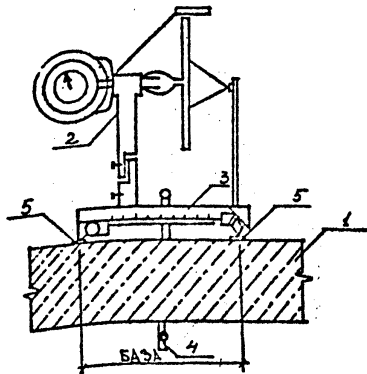
ЭЛЕКТРОМЕХАНИЧЕСКИЙ ТЕНЗОМЕТР АИСТОВА
