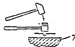
Нанесение удара обычным молотком по головке эталонного молотка
