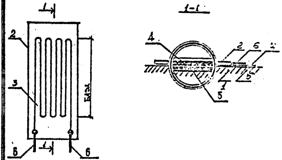
ТЕНЗОРЕЗИСТОР
