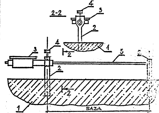
ИНДИКАТОР ЧАСОВОГО ТИПА
