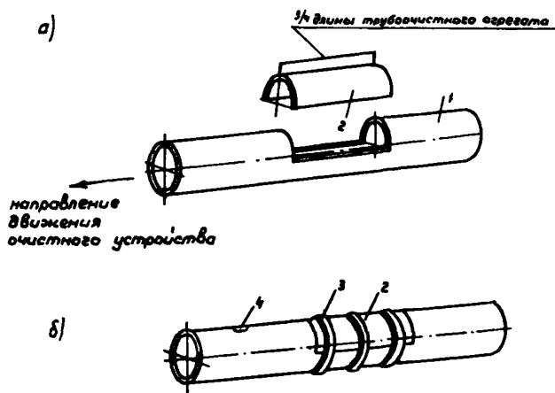
Рис.5 а) камера пуска очистного агрегата; б) устройство герметизации камер: 1 - трубопровод; 2 - крышка камер; 3 - бандаж; 4 - заглушка.
