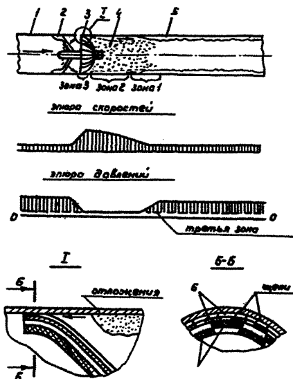
Рис.3. Гидродинамическое очистное устройство
