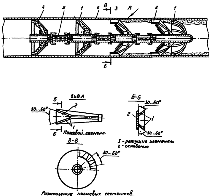
Рис.1. Гидромеханическое очистное устройства
