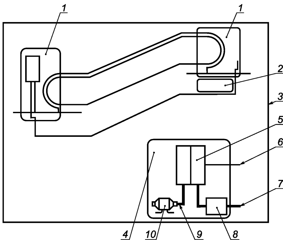
Рисунок 2 — Вариант представления эскалатора и пассажирского конвейера в виде системы (помехозмиссия)
