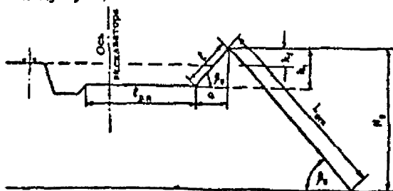
Рис. 2.1. Схема поверхности отвала при отвалообразовании мехлоплатой
