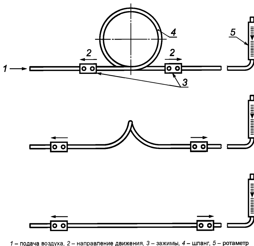
Рисунок 3 – Испытания шланга подачи сжатого воздуха на деформацию
