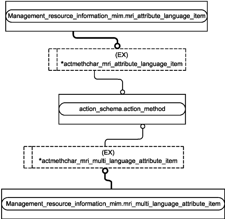
Рисунок D.6 — Представление ИММ на уровне объектов в формате EXPRESS-G (диаграмма 5 из 5)
