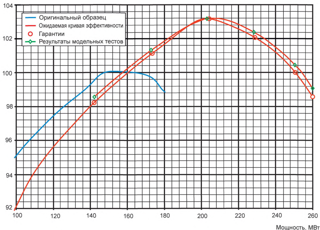
Рисунок 4 — Сравнительная эффективность по сравнению с первоначальной производительностью — Первоначальные и новые рабочие колеса — генерирующая станция Outrades 3
