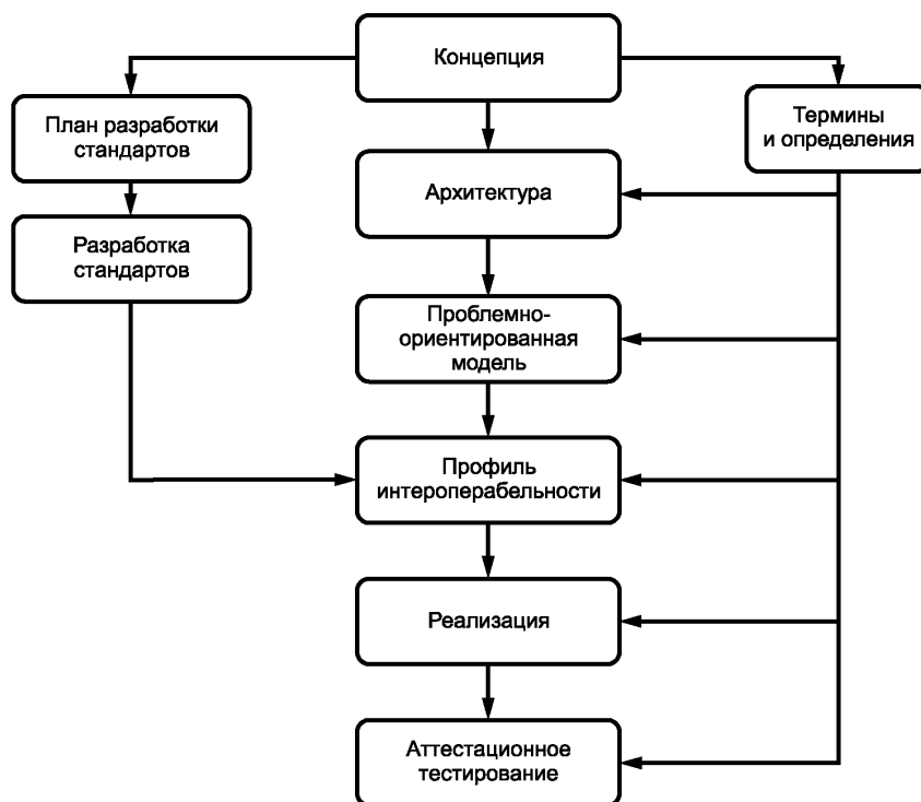
Рисунок 2 — Основные этапы обеспечения интероперабельности
