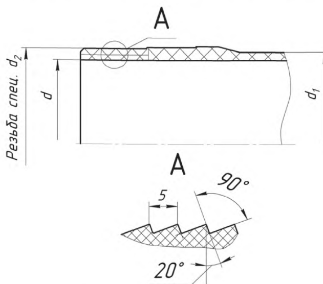
d – внутренний диаметр трубы; d_1 – наружный диаметр трубы; d_2 – диаметр ниппеля Рисунок 3 – Ниппель под соединение «KPS»
